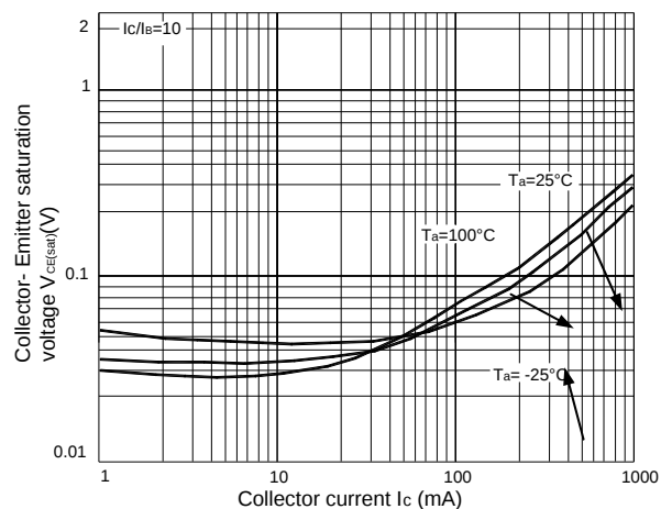
Fig. 4 V_{CE(sat)} - I_c
