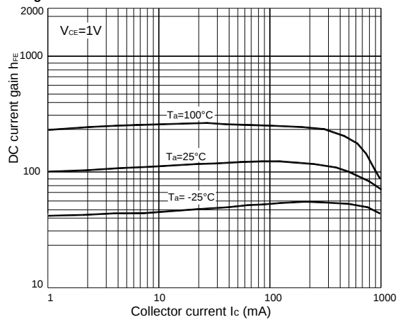
Fig.5 h_{FE} - I_c
